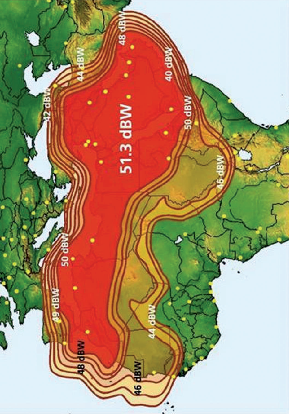
مجال تغطية ساتل بدر 5 (arabe-pan-ku)
